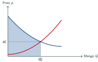
Nutzen
