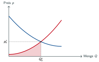
Variable Kosten
